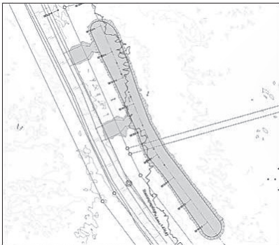
Abbildung: Planung SAG-Ingenieure GmbH - Variante 4
