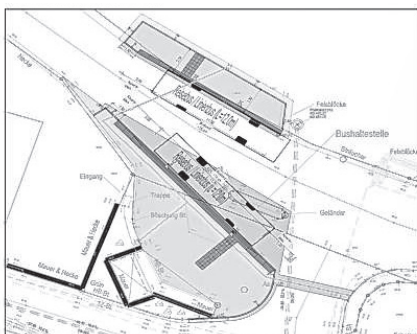
Abbildung: Planung Kling Consult GmbH - barrierefreie Bushaltestellen Neuhausen
